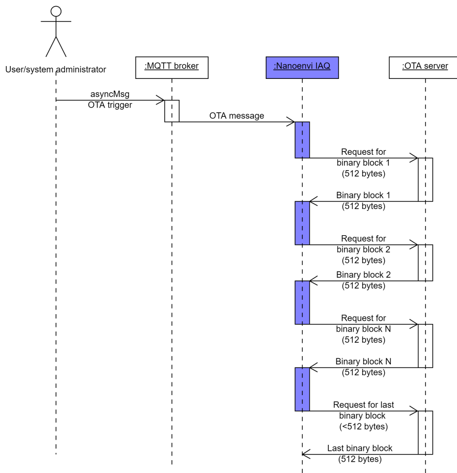
Diagrama de secuencia de actualización OTA
